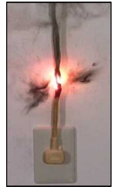
(写真) 不適切な修理によって異常発熱・発火したエアコンの電源コード
